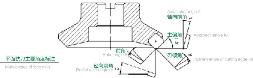
平面铣刀主要角度标注 Main Angles of Face Mill
